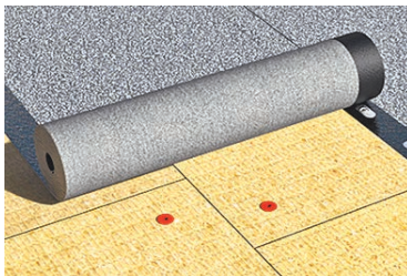
Рис. 3. Однослойный кровельный материал двойного крепления.
