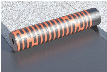
Рис. 4. Битумно-полимерный материал с системой вентиляции.
