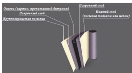
Рис. 2. Структура рулонных кровельных материалов.
